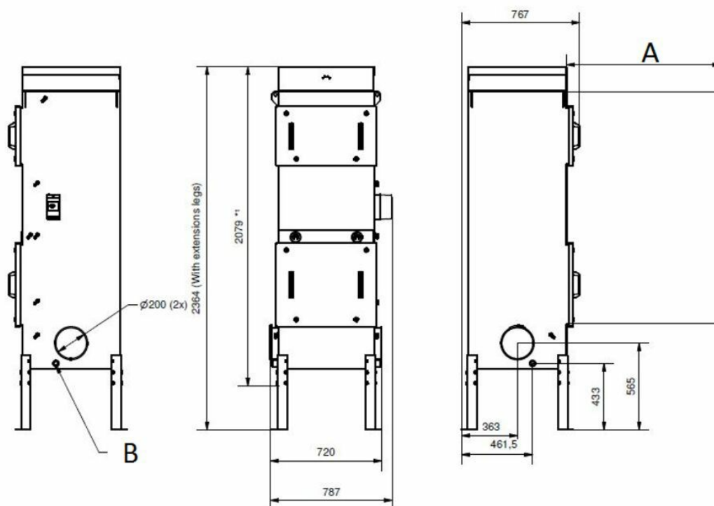
A) 1000mm proctor pro servis filtrů B) Drenáž (x2)
